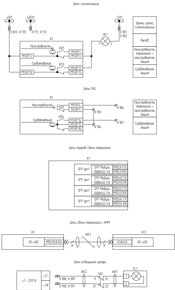
Рисунок В.5 – Схема электрическая принципиальная (часть 5)
